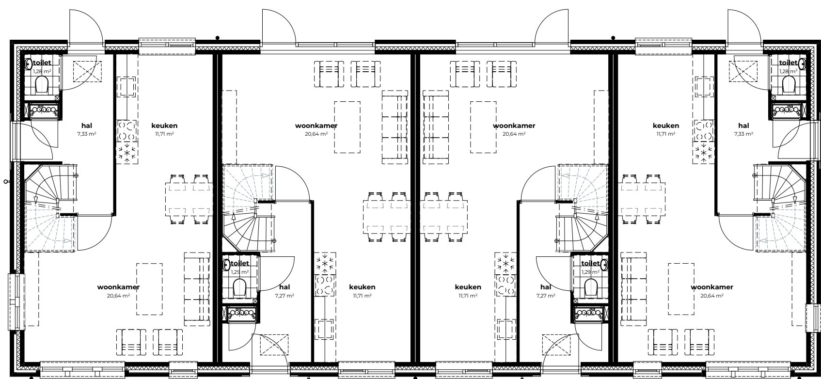
Rijwoningen - Begane grond
