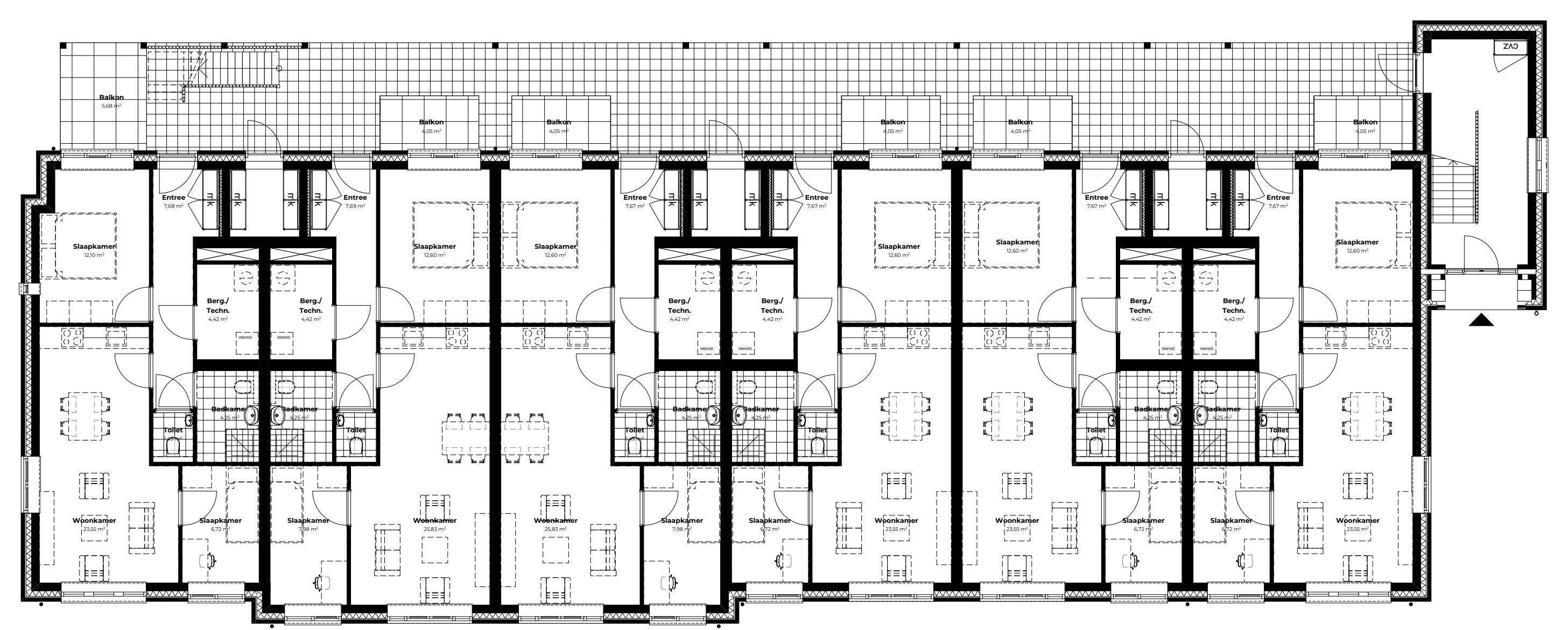
Appartementen Thomaslaan - Begane grond (eerste etage identiek)
