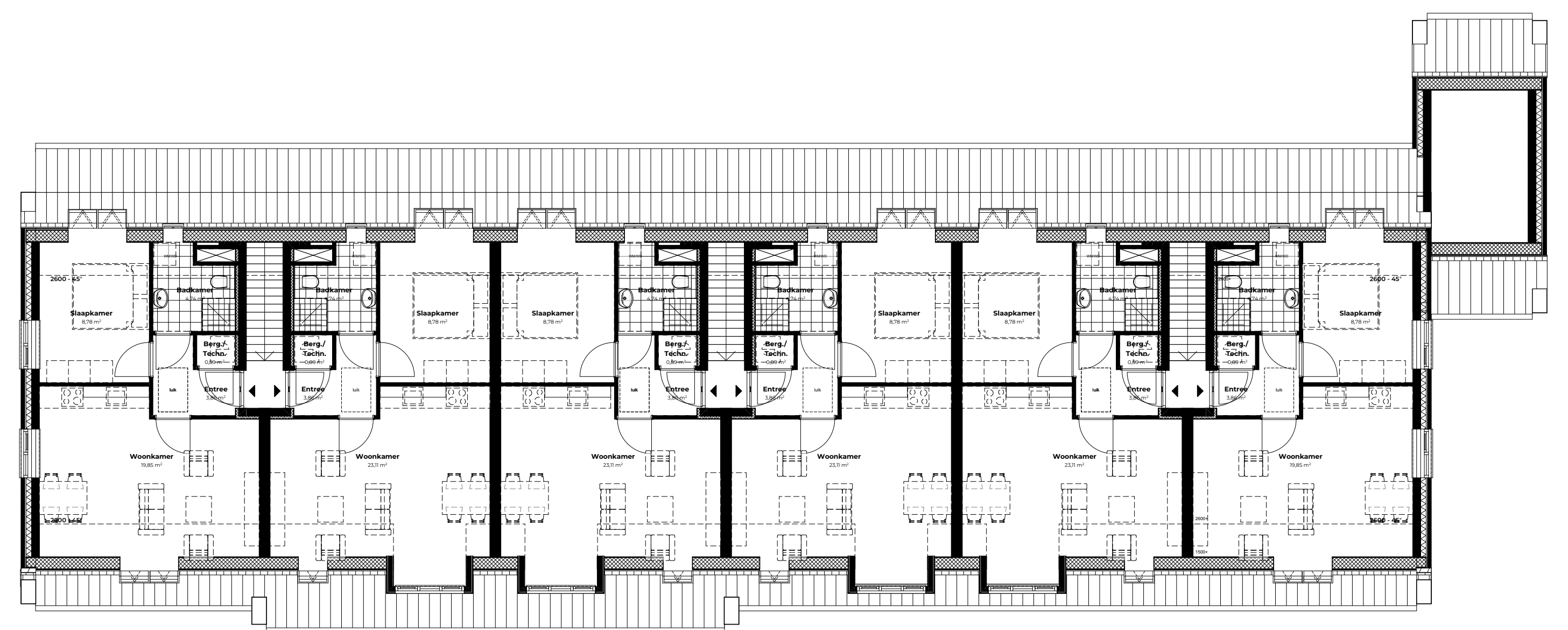
Appartementen Thomaslaan - Tweede verdieping
