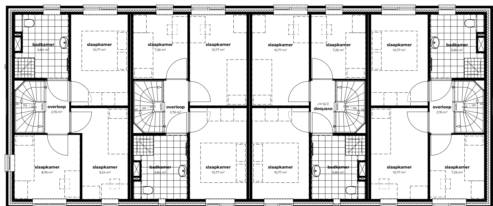
Rijwoningen - Eerste verdieping
