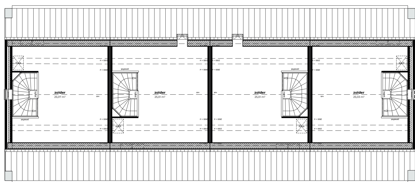
Rijwoningen - Tweede verdieping
