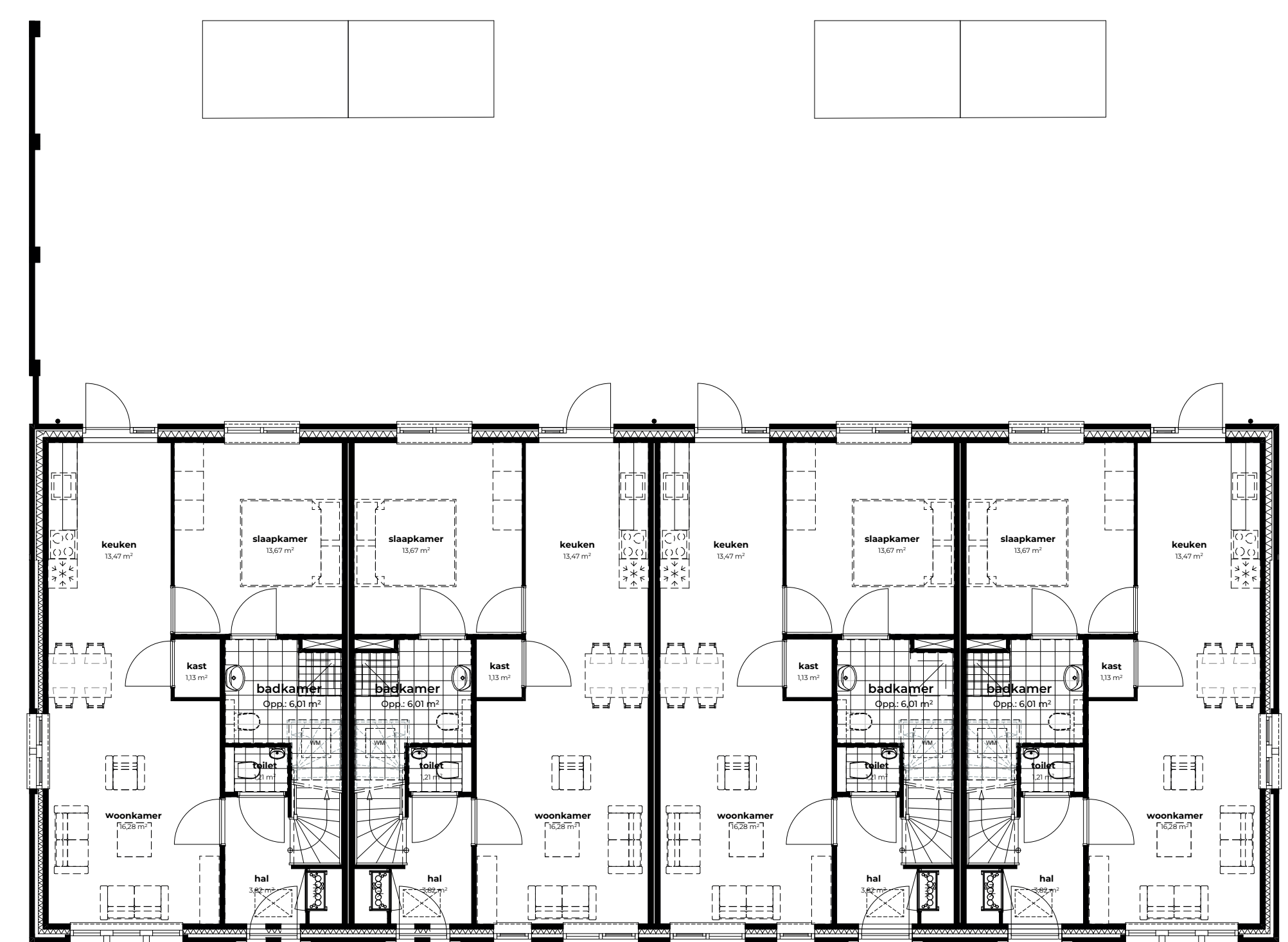
Levensloopwoningen - Begane grond
