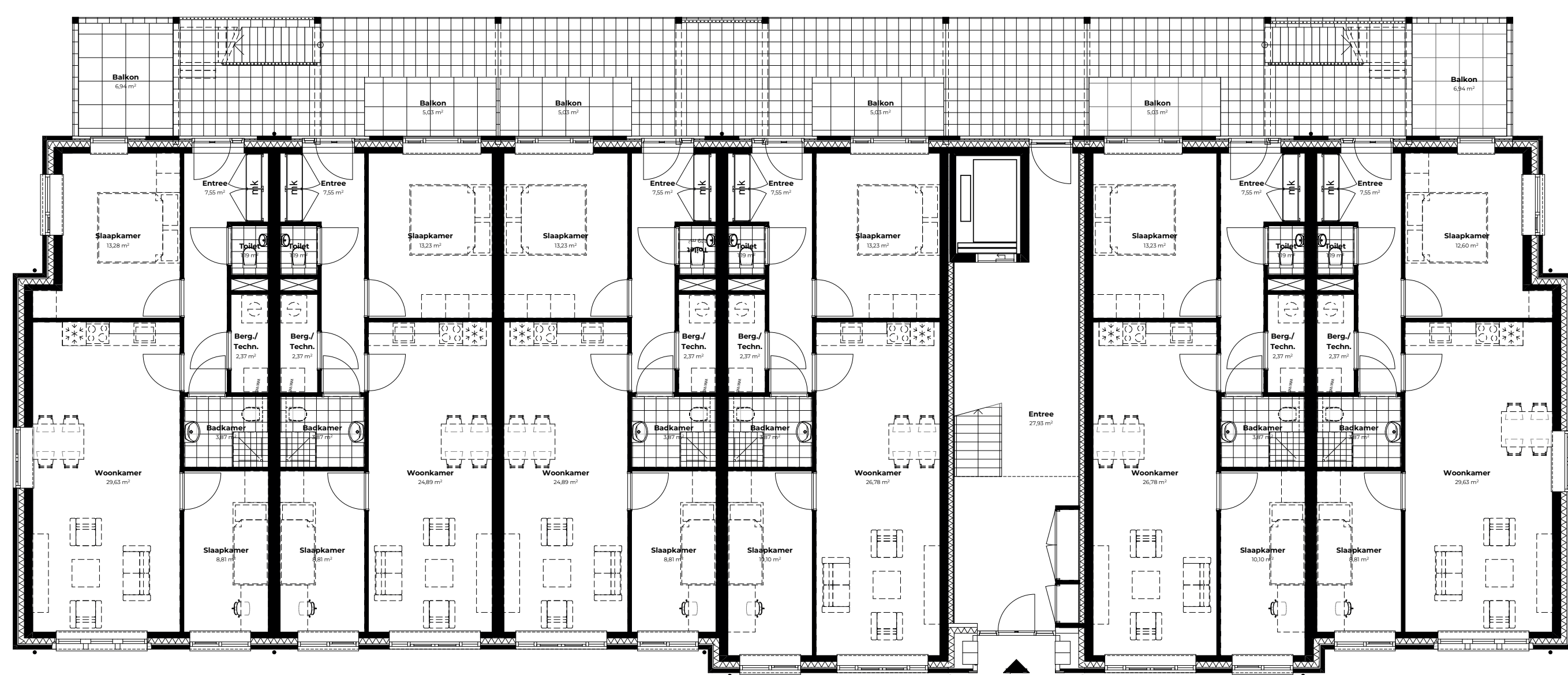
Appartementen Van Voorhuizenlaan - Begane grond (eerste etage identiek)
