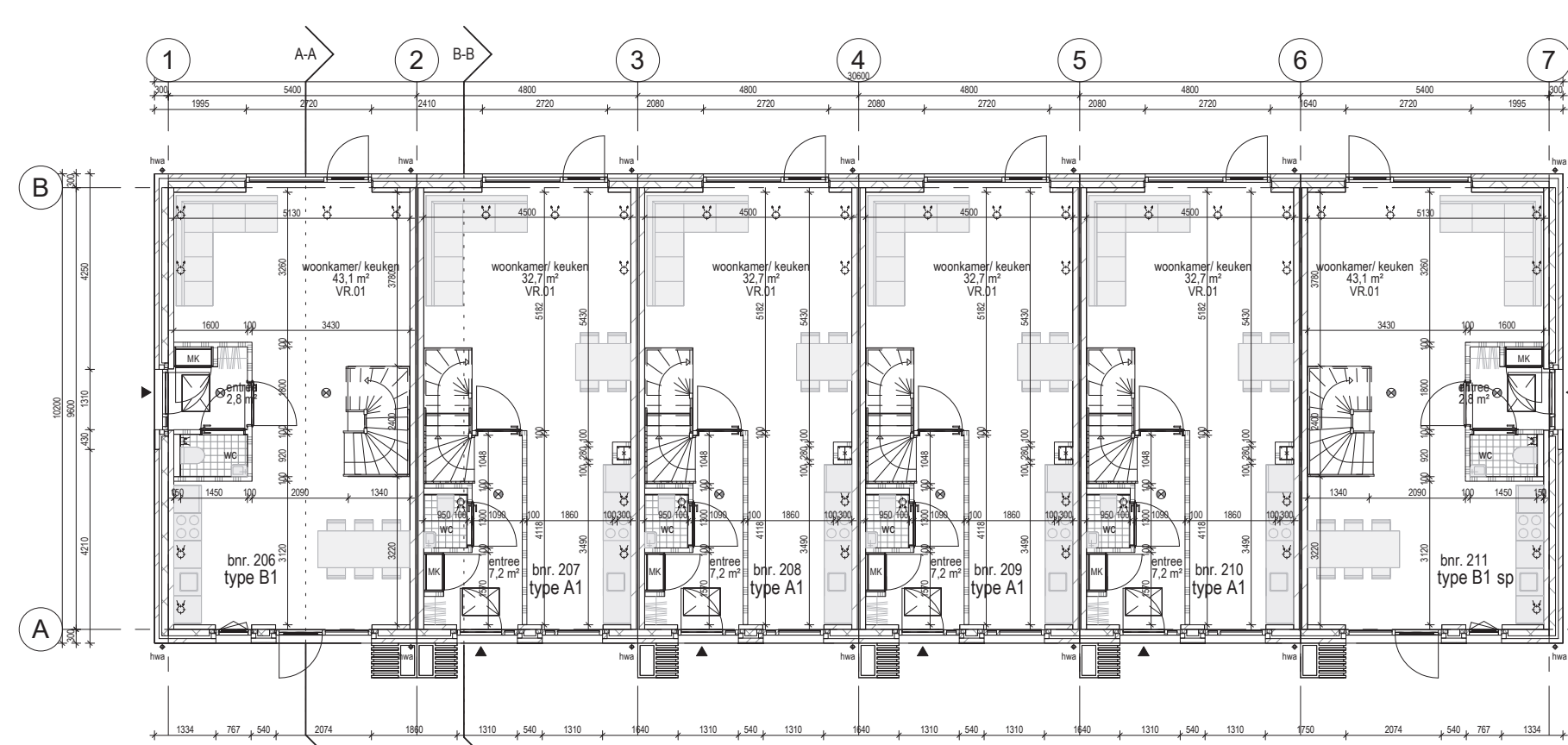
Begane grond KA -> blok KC=KA, uitzondering kopwoningen zijn 5100mm
