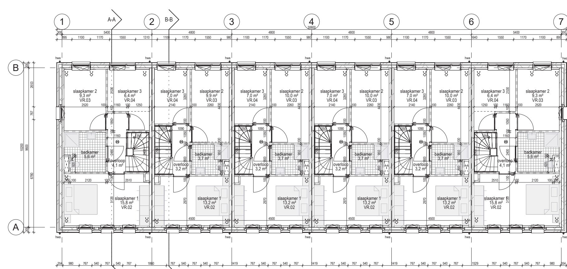
1e verdieping KA
