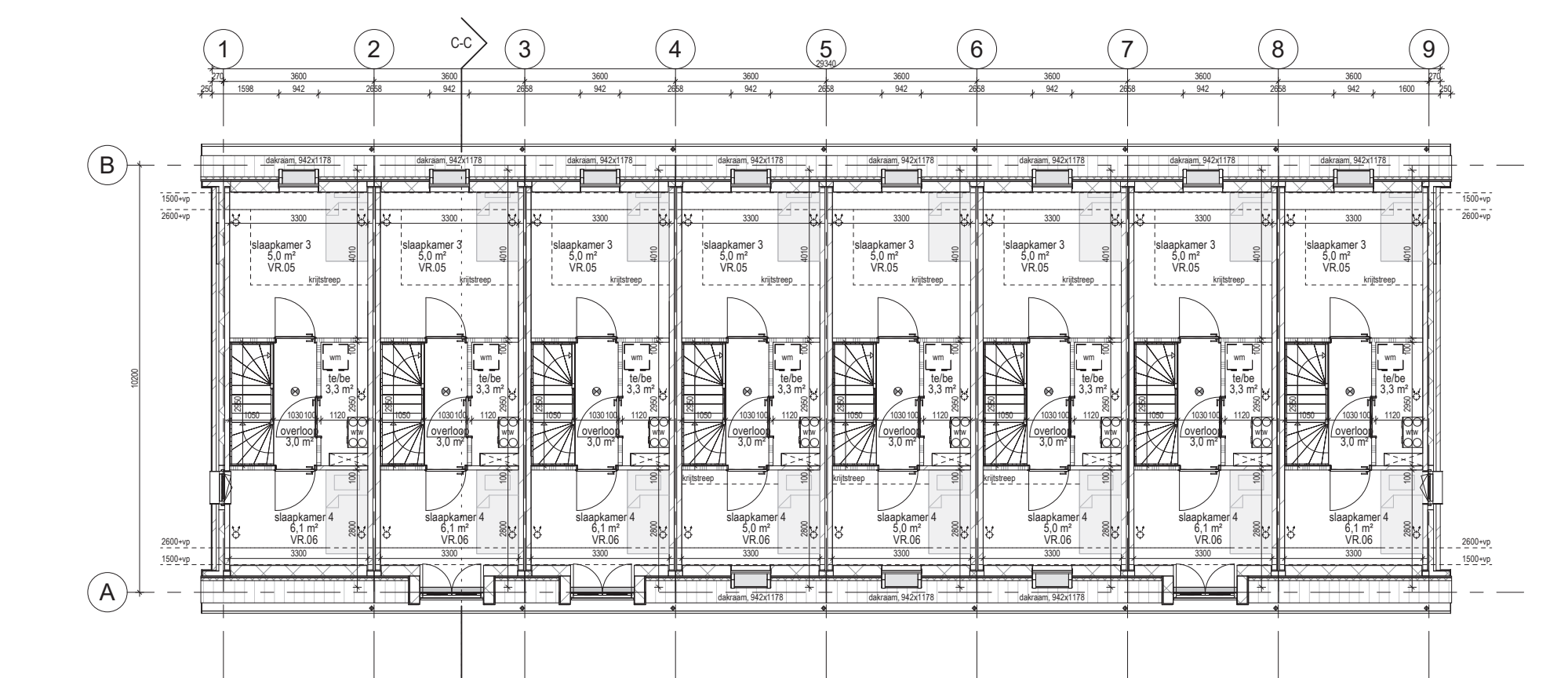
2e verdieping KB
