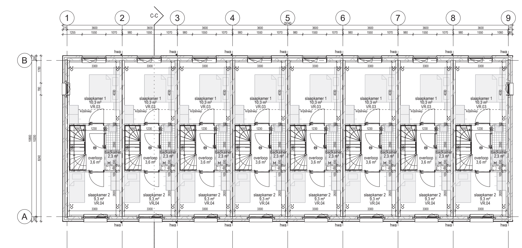
1e verdieping KB
