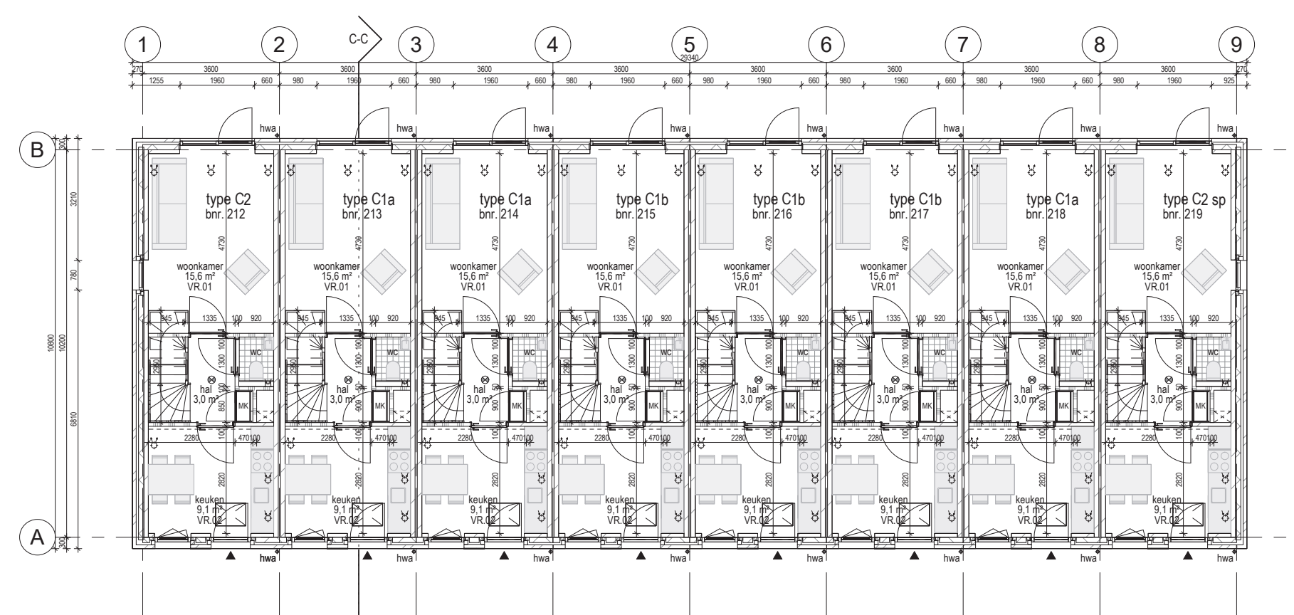
Begane grond KB
